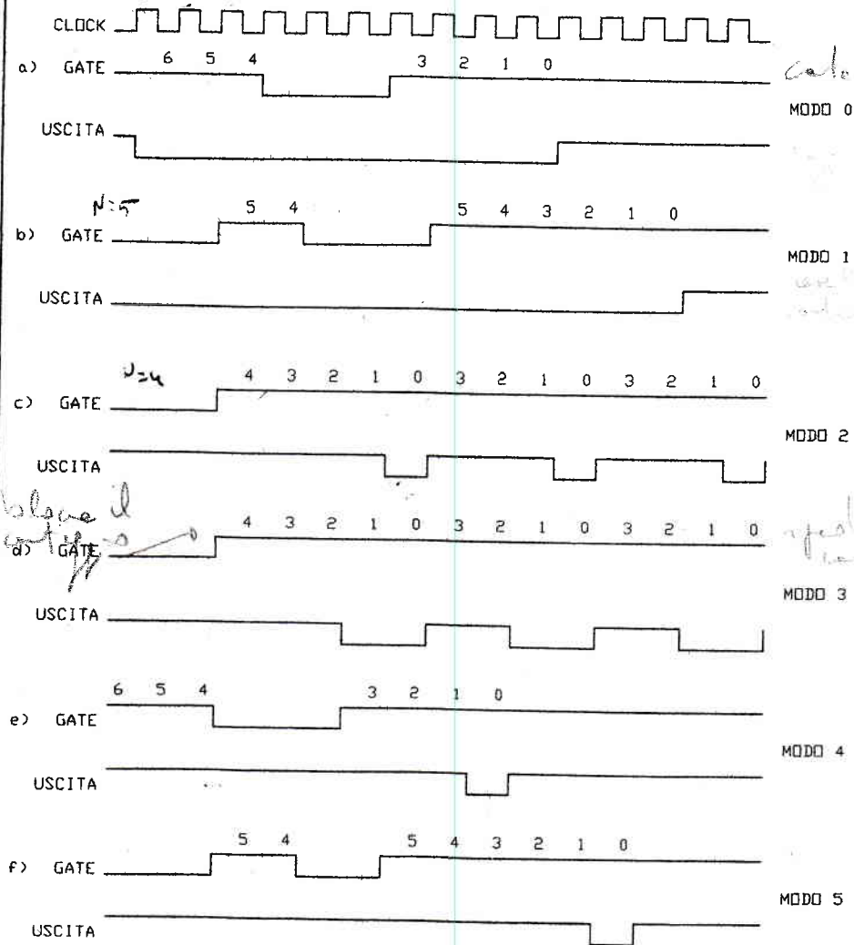
Fig. B.3 - diagrammi di temporizzazione per i sei modi di funzionamento dell'INTEL 8253 a) modo 0 d) modo 3 b) modo 1 e) modo 4 c) modo 2 f) modo 5
